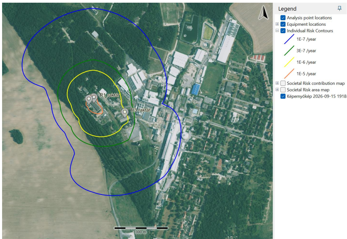
Az Agroterm Kft. egyéni kockázati görbéi tűz hőterhelés hatásra
