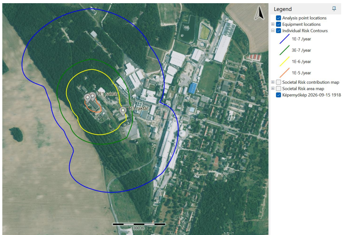
Az Agroterm Kft. egyéni kockázati görbéi toxikus hatásra
